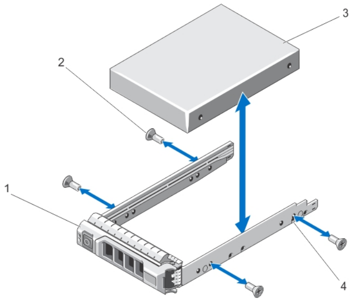
Ilustración 23. Extracción e instalación de una unidad de disco duro de intercambio activo en un portaunidades de disco duro
