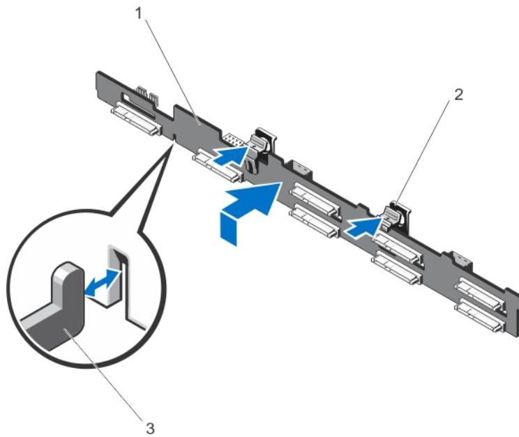
Ilustración 50. Extracción e instalación del plano posterior de ocho unidades de disco duro
