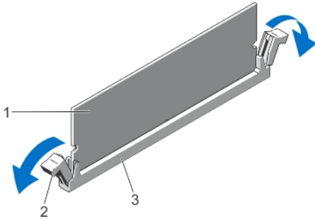
Ilustración 15. Expulsión del módulo de memoria
