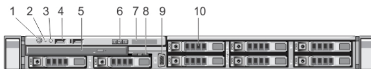
Ilustración 2. Características e indicadores del panel frontal: sistema con ocho unidades de disco duro de 2,5 pulgadas
