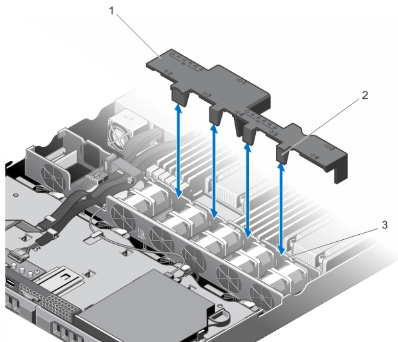
Ilustración 13. Extracción e instalación de la cubierta de refrigeración
