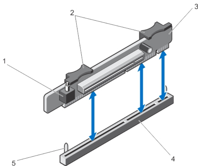
Ilustración 33. Extracción e instalación del soporte vertical de tarjeta de expansión 2
