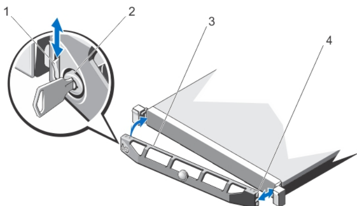
Ilustración 9. Instalación y extracción del embellecedor frontal
