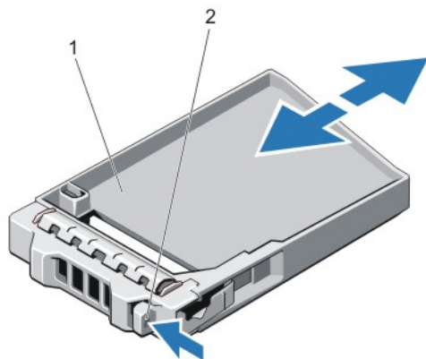
Ilustración 18. Extracción e instalación de una unidad de disco duro de relleno de 2,5 pulgadas
