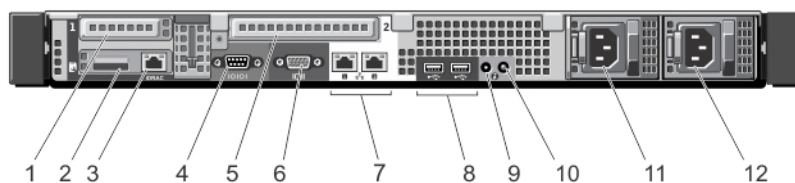
Ilustración 6. Características e indicadores del panel posterior
