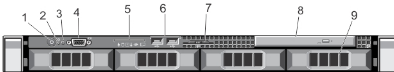
Ilustración 3. Características e indicadores del panel frontal: sistema con unidad de disco duro cableado de 3,5 pulgadas
