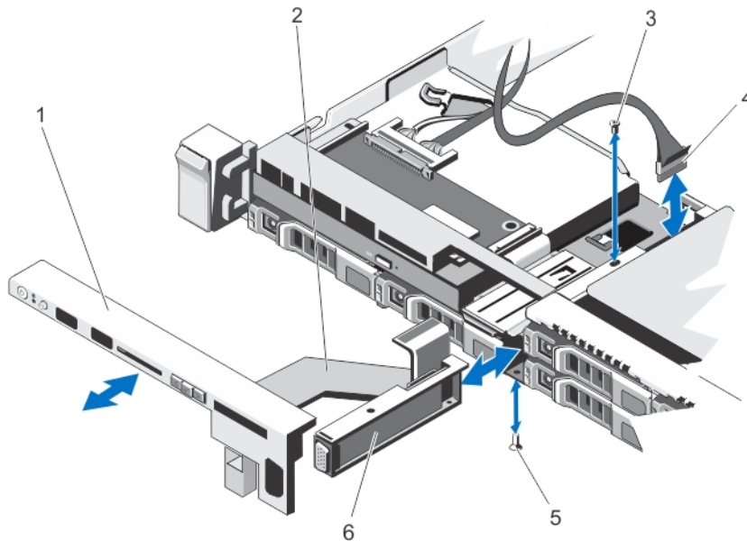
Ilustración 57. Extracción e instalación del módulo VGA
