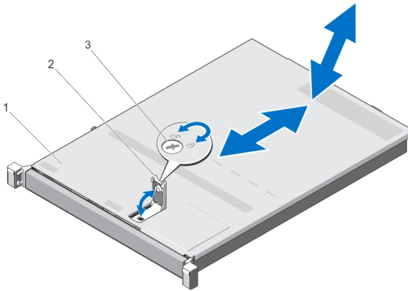
Ilustración 10. Apertura y cierre del sistema
