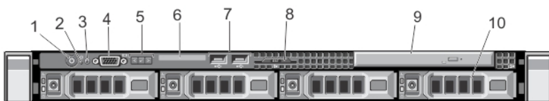
Ilustración 1. Características e indicadores del panel frontal: sistema con unidad de disco duro de 3,5 pulgadas
