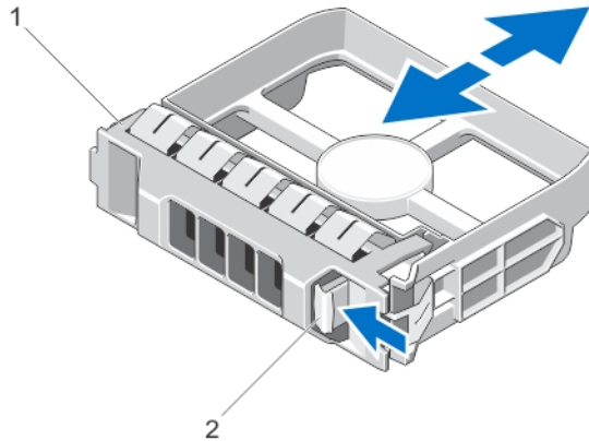
Ilustración 19. Extracción de una unidad de disco duro de relleno de 3,5 pulgadas
