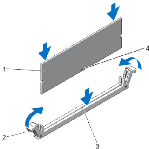
Ilustración 17. Instalación del módulo de memoria
