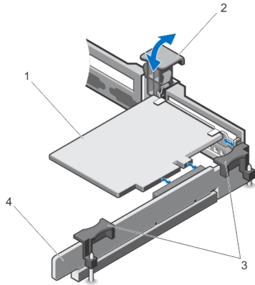
Ilustración 30. Extracción e instalación de la tarjeta de expansión del soporte vertical de tarjeta de expansión 1
