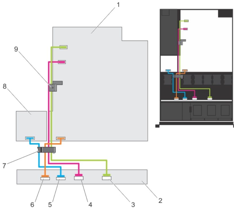
Ilustración 51. Diagrama del cableado: plano posterior de ocho unidades de disco duro
