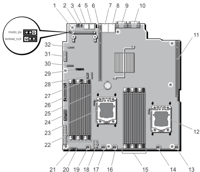
Ilustración 61. Puentes y conectores de la placa base
