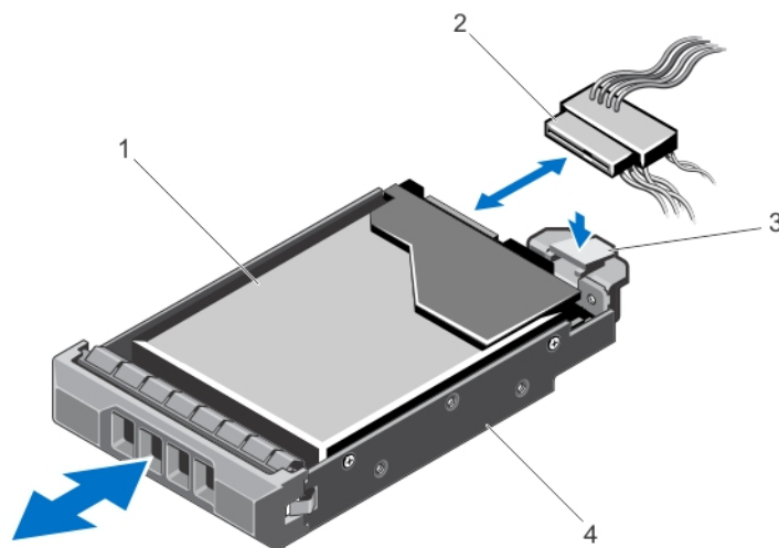
Ilustración 21. Extracción e instalación de una unidad de disco duro cableado
