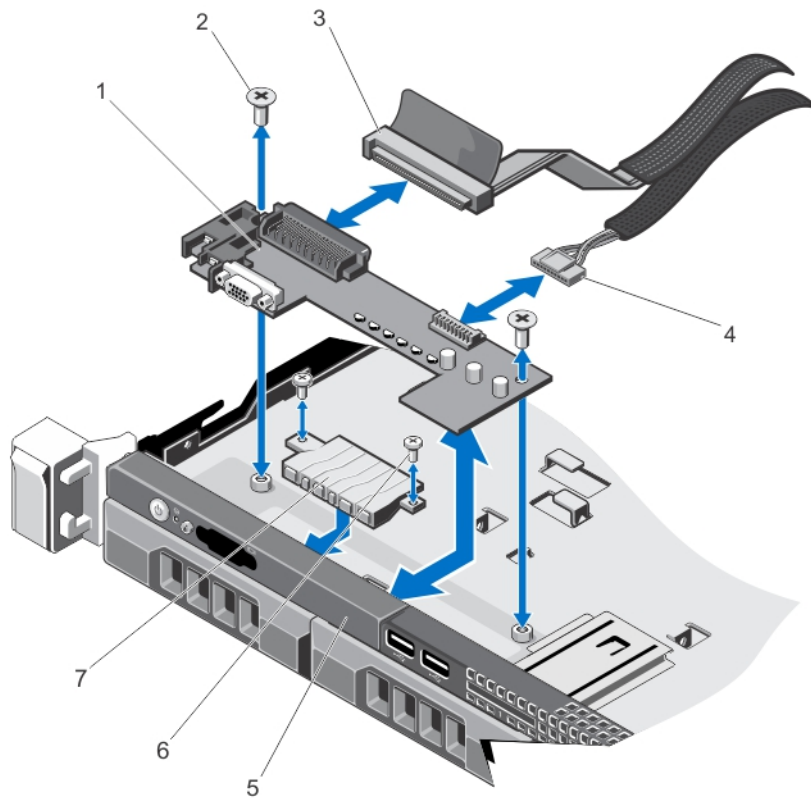
Ilustración 54. Extracción e instalación del módulo del panel de control: sistemas con unidad de disco duro cableado de 3,5 pulgadas
