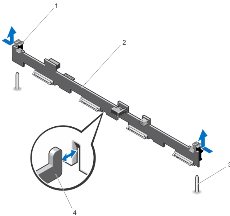
Ilustración 46. Extracción e instalación del plano posterior de cuatro unidades de disco duro
