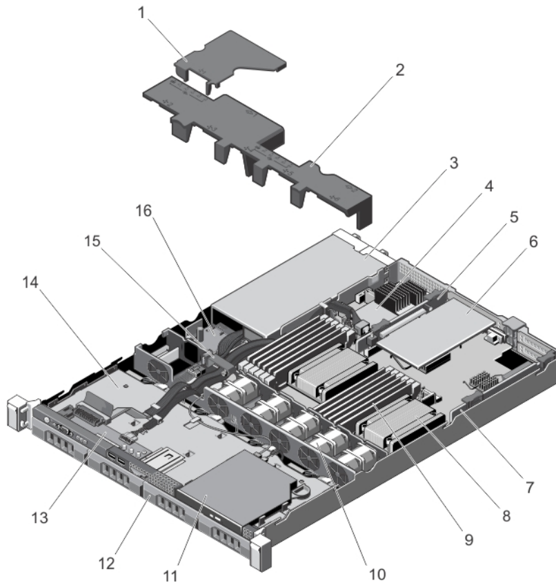
Ilustración 12. Interior del sistema: con fuentes de alimentación redundantes
