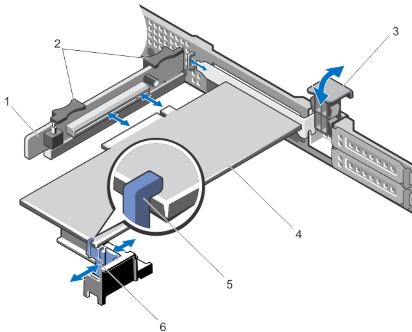
Ilustración 31. Extracción e instalación de la tarjeta de expansión del soporte vertical de tarjeta de expansión 2
