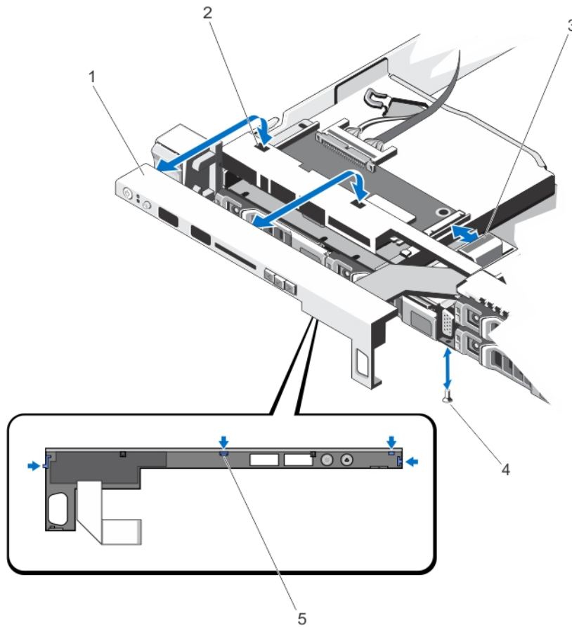
Ilustración 53. Extracción e instalación del panel de control: sistemas con ocho unidades de disco duro
