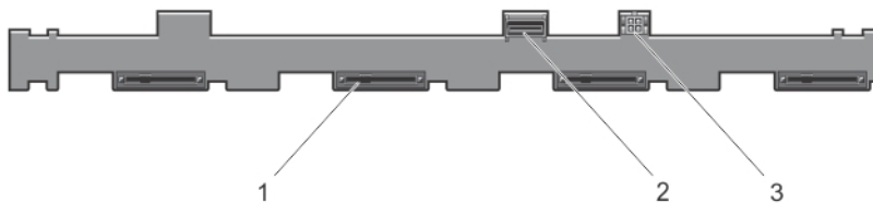
Ilustración 44. Vista frontal del plano posterior de cuatro unidades de disco duro
