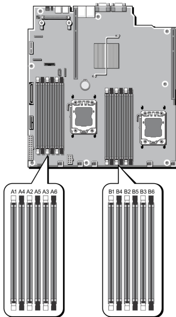
Ilustración 14. Ubicación de los zócalos de memoria
