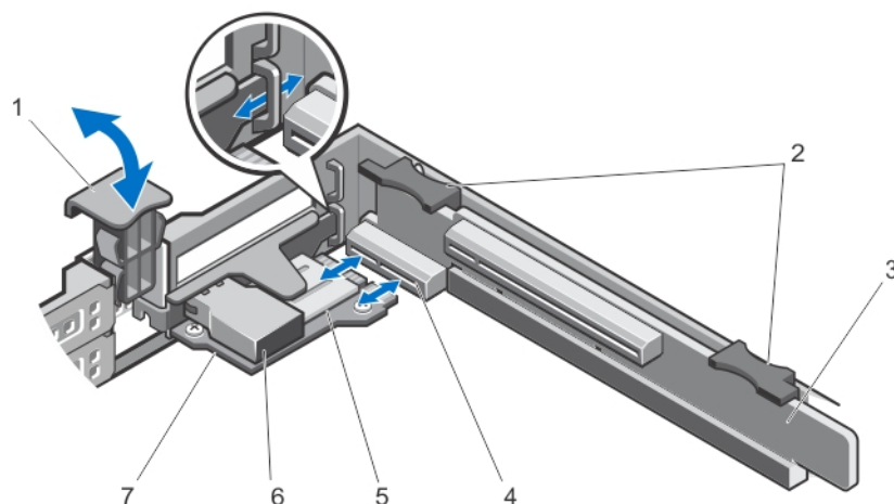
Ilustración 34. Extracción e instalación de la tarjeta de puertos iDRAC
