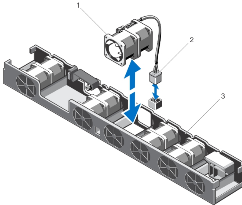
Ilustración 28. Extracción e instalación de un ventilador de refrigeración
