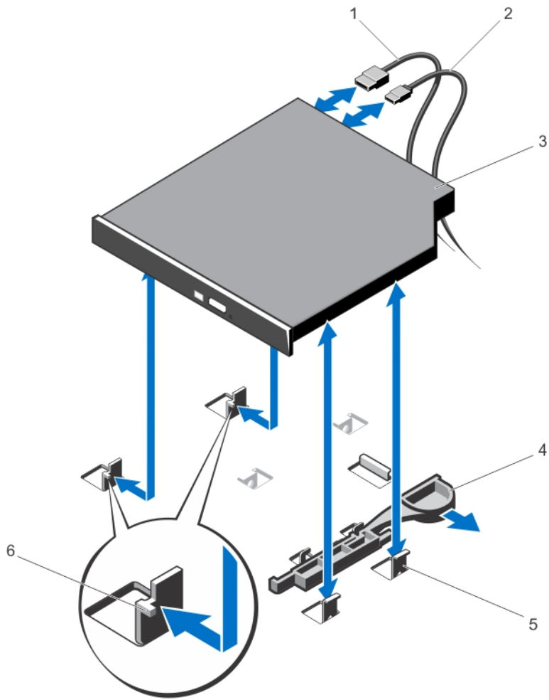
Ilustración 27. Extracción e instalación de la unidad óptica (sistemas con unidad de disco duro cableado)
