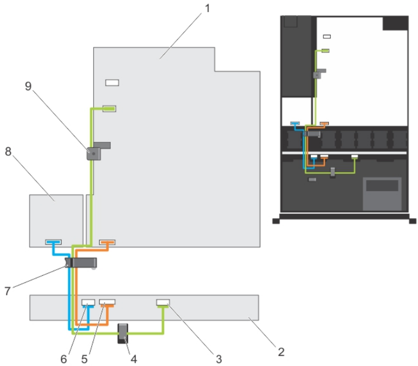
Ilustración 47. Diagrama del cableado: plano posterior de cuatro unidades de disco duro
