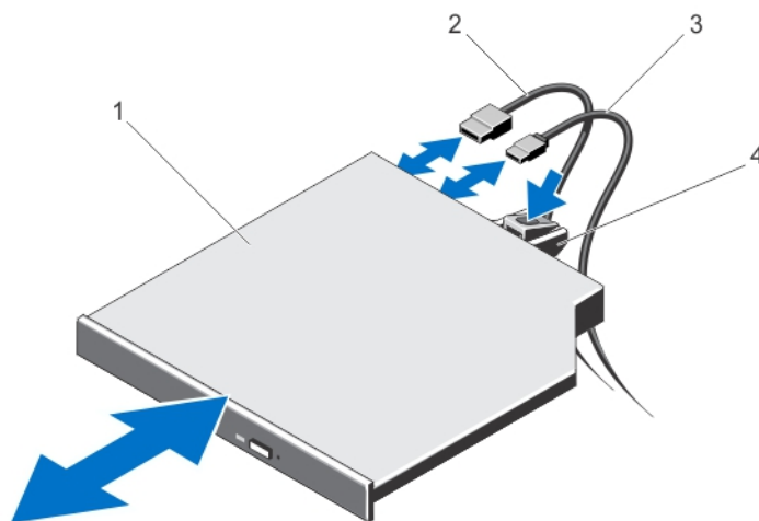
Ilustración 26. Extracción e instalación de la unidad óptica (sistemas con unidad de disco duro de intercambio activo)
