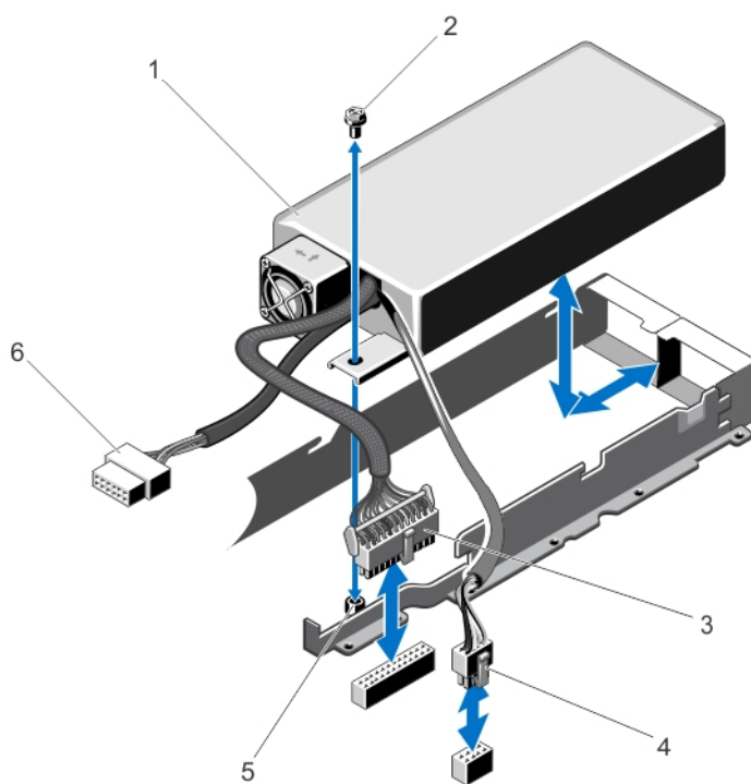
Ilustración 41. Extracción e instalación de un fuente de alimentación no redundante
